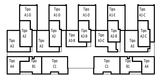
PLANTA PISOS 3-4
