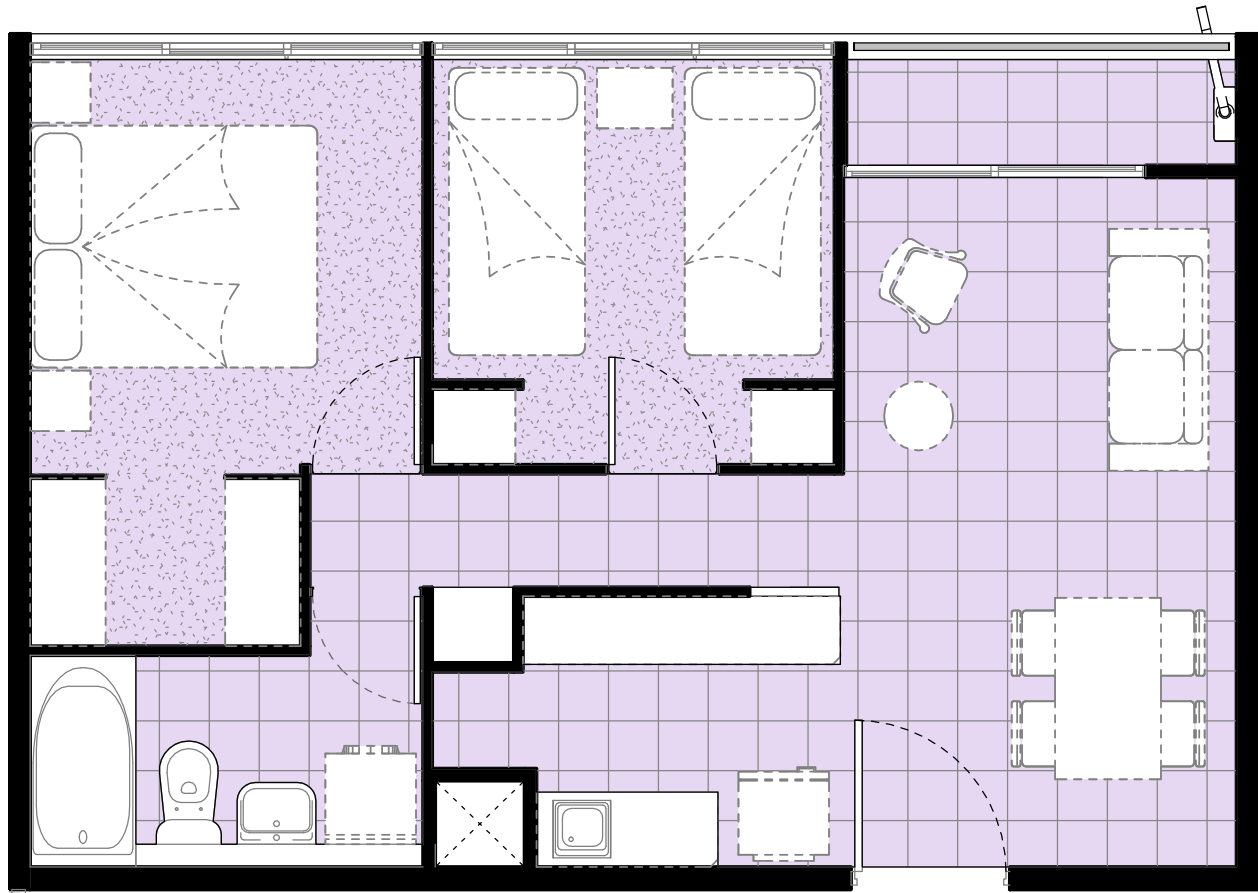
DEPARTAMENTO TIPO 2D+1B
